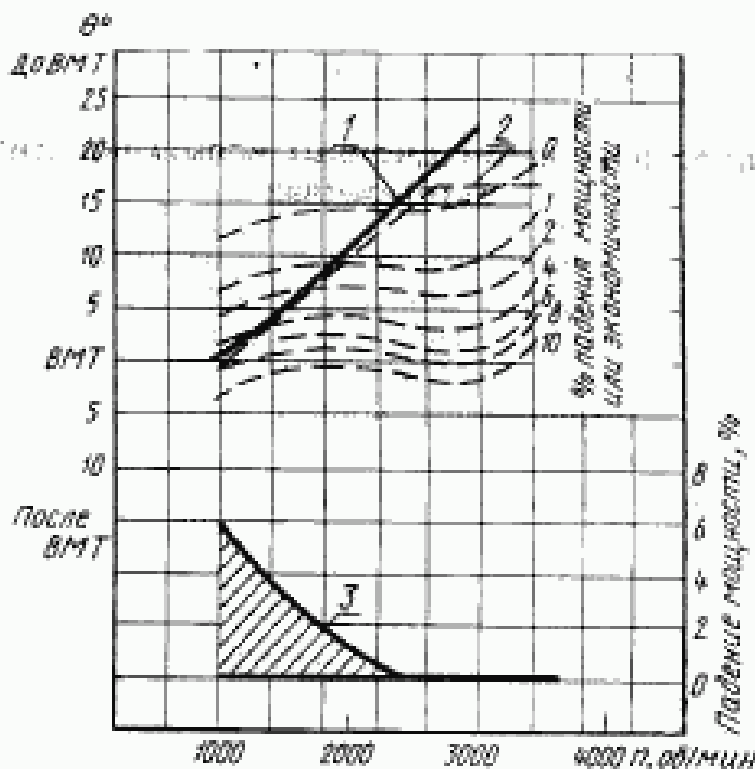
1—детонационная характеристика заданного бензина; 2—выбранная характеристика автомата; 3—линии мощ- ности
